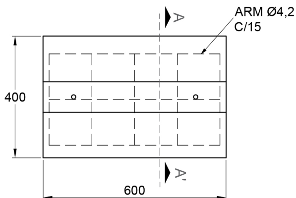
PLANTA -PUNTERA 400 X 600 mm
