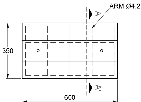
PLANTA -PUNTERA 350 X 600 mm
