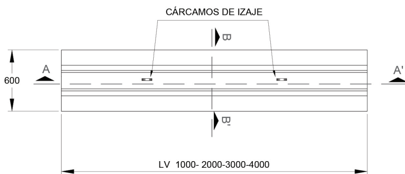
PLANTA - DEFENSA LV - H= 800 m
