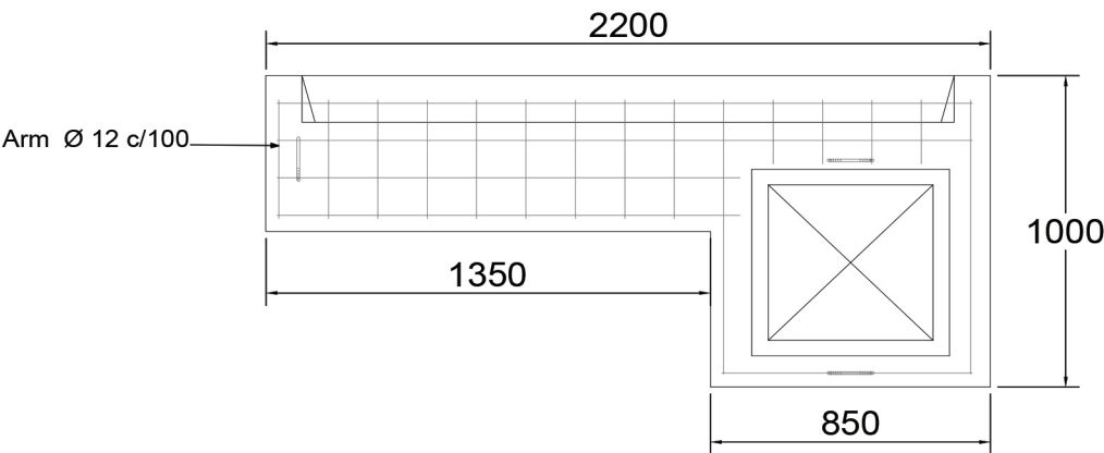
TAPA SUMIDERO
