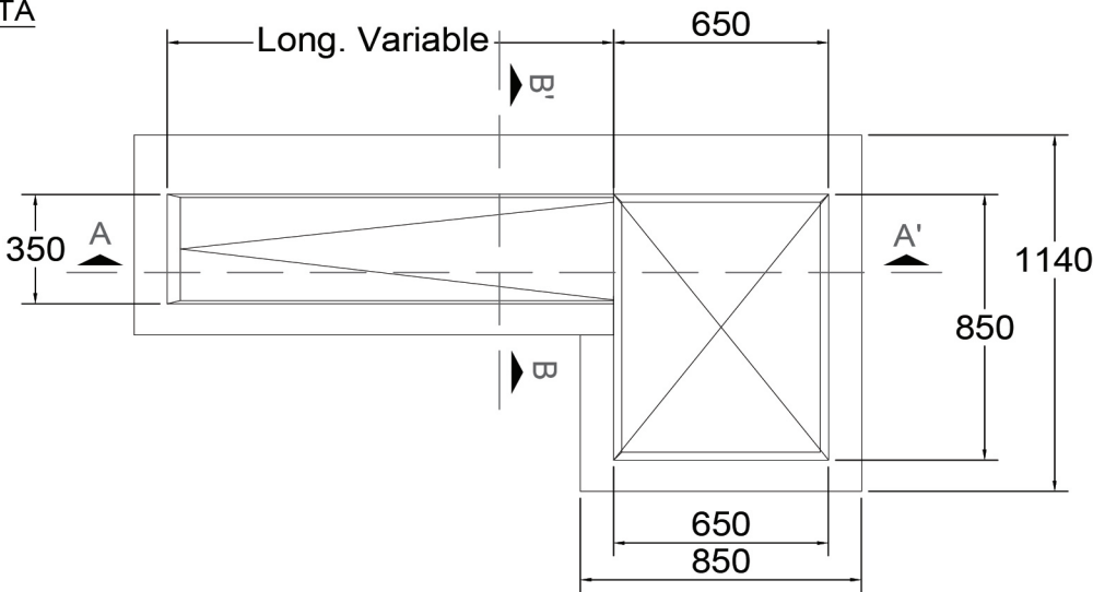
TAPA SUMIDERO
