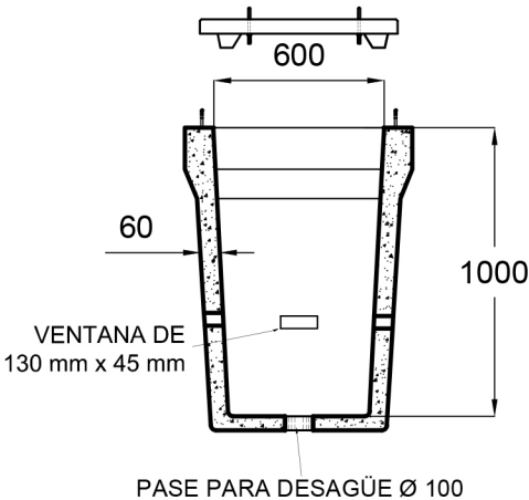
CORTE B -B' - CÁMARA A0
