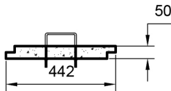
CORTE C-C' TAPA D2P
