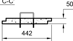
CORTE C-C'
