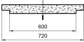
CORTE B-B'
