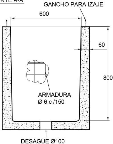
CORTE A-A'
