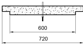
CORTE B-B'
