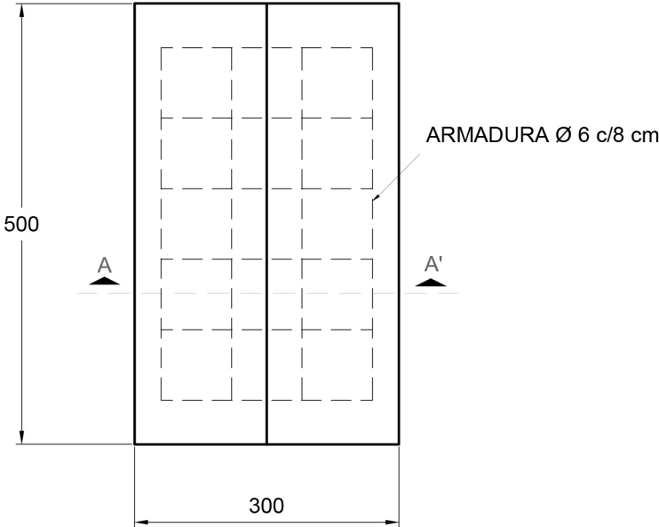
CORTE A-A'
