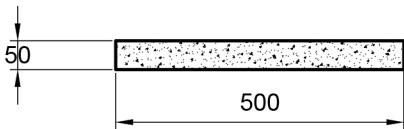
CORTE A-A' - LOSA CUBRECABLES 132 KV - Sin armadura
