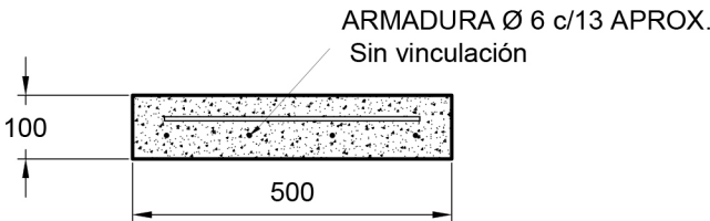
CORTE A-A' - LOSA CUBRECABLES 132 KV - Con armadura
