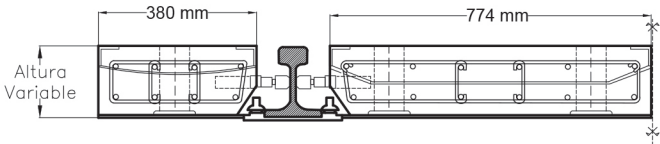
CORTE A-A' - LOSAS PASO NIVEL L - C
